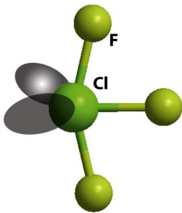
3 ClF 3 , C 2v
